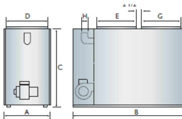
BFL : COLLECTEUR COMBINÉ AVANT
