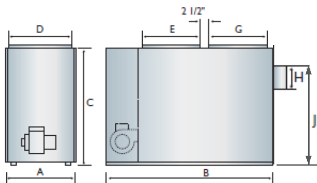
BCL-S : COLLECTEUR COMBINÉ ARRIÈRE
