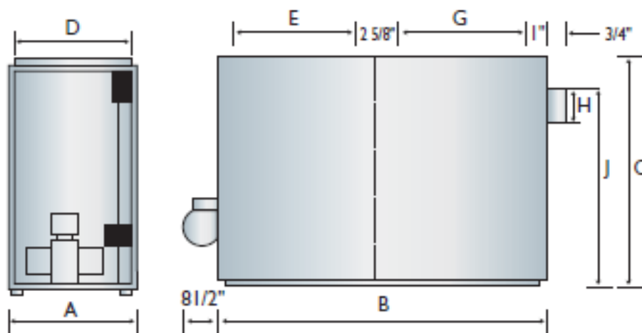
BCL 190/225 haute capacité COLLECTEUR COMBINÉ ARRIÈRE
