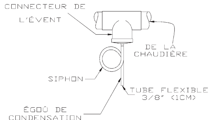
Figure 11 - Système De Collection De Condensats
